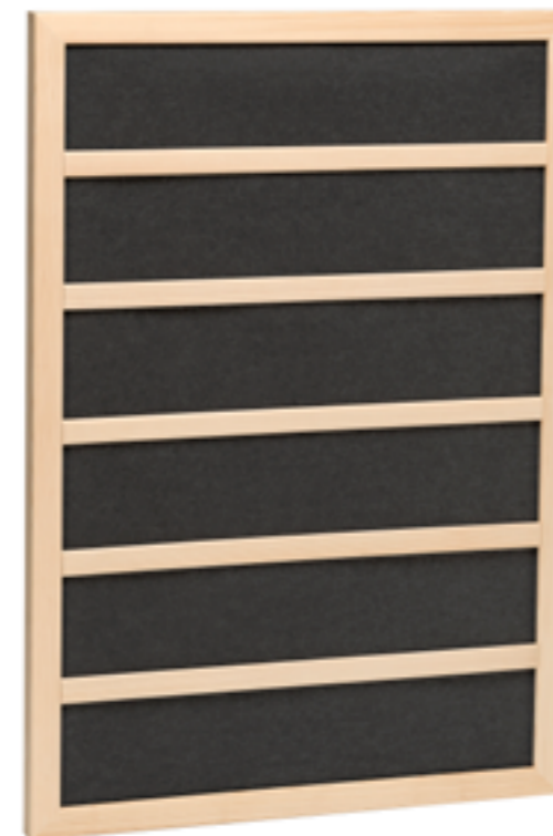
Puissance : 300 W 680 (l) x 37 (p) x 980 (h) mm
