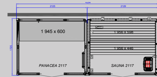
TWIN PANACEA 2117 Dimensions : (p) 2 125 x (l) 4 254 mm
