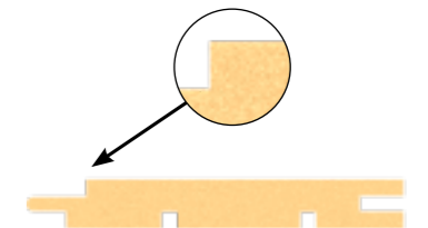
2. PROFILÉ STS DE PANNEAU DE SAUNA
