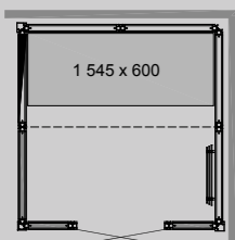
PANACEA 1717 1B Dimensions : 1 725 x 1 725 x 2 090 mm
