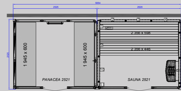
TWIN PANACEA 2521 Dimensions : (p) 2 125 x (l) 5 054 mm
