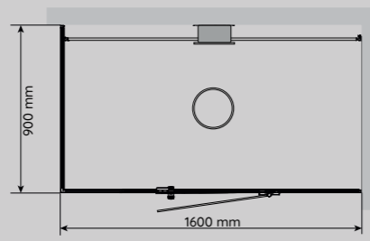
VISTA 160 À DROITE Dimensions : (p) 900 x (l) 1 600 mm
