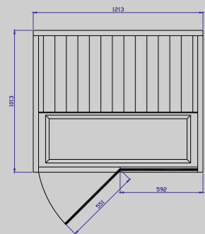
TYLÖSAND T-820 Dimensions : (p) 1 013 mm x (l) 1 213 mm Puissance : 1 470 W
