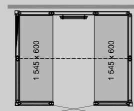
PANACEA 2117 2B Dimensions : 2 125 x 1 725 x 2 090 mm
