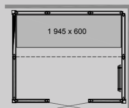
PANACEA 2117 1B Dimensions : 2 125 x 1 725 x 2 090 mm
