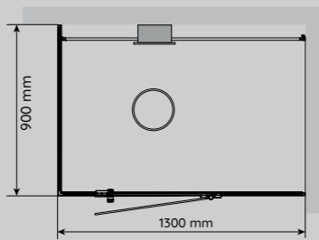
VISTA 130 À GAUCHE Dimensions : (p) 900 mm x (l) 1 300 mm
