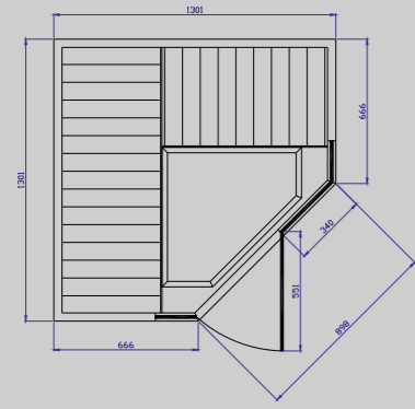
TYLÖSAND T-870 Dimensions : (p) 1 301 x (l) 1 301 mm Puissance : 1 600 W
