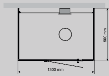
VISTA DCO 130 À DROITE Dimensions : (p) 900 mm x (l) 1 300 mm
