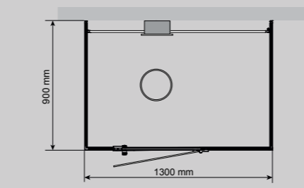
VISTA DCO 130 À GAUCHE Dimensions : (p) 900 x (l) 1 300 mm
