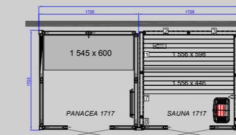
TWIN PANACEA 1717 Dimensions : (p) 1 725 x (l) 3 454 mm
