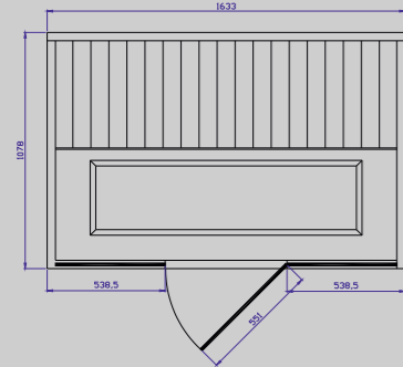
TYLÖSAND T-825 Dimensions : (p) 1 078 x (l) 1 633 Puissance : 1 980 W
