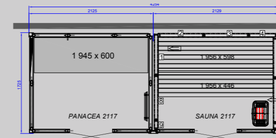
TWIN PANACEA 2117 Dimensions : (p) 2 125 x (l) 4 254 mm
