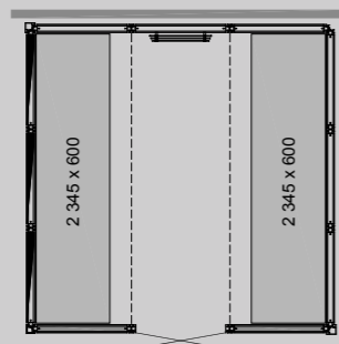
PANACEA 2525 2B Dimensions : 2 525 x 2 525 x 2 090 mm
