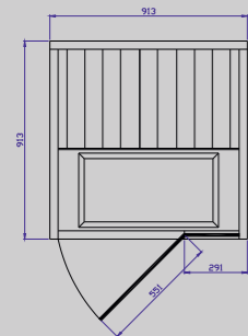
TYLÖSAND T-810 Dimensions : (p) 913 mm x (l) 913 mm Puissance : 1350W
