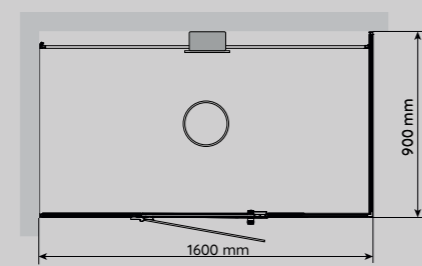
VISTA 160 À DROITE Dimensions : (p) 900 mm x (l) 1 300 mm
