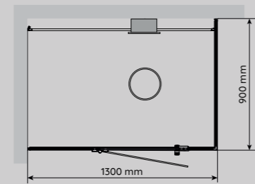
VISTA 130 À DROITE Dimensions : (p) 900 mm x (l) 1 300 mm
