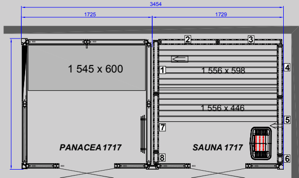
TWIN PANACEA 1717 Taille : 1 725 mm (p) x 3 454 mm (l)
