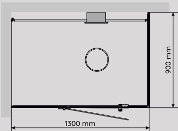
VISTA 130 DROITE Taille : 900 mm (p) x 1 300 mm (l)
