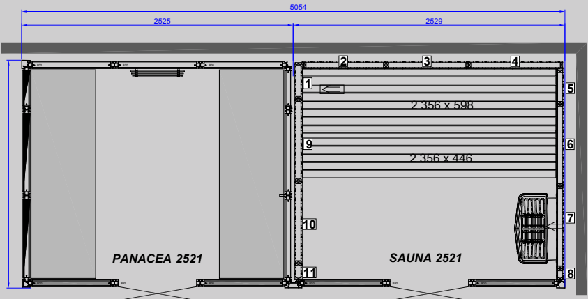
TWIN PANACEA 2521 Taille : 2 125 mm (p) x 5 054 mm (l)
