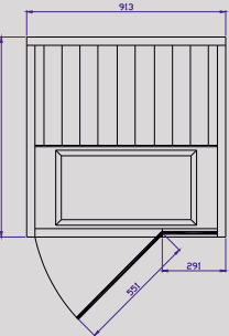
TYLÖSAND T-810 Taille : 913 mm (p) x 913 mm (l) Power : 1350W
