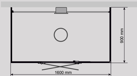
VISTA DCO 160 (GAUCHE ET DROITE) Taille : 900 mm (p) x 1 600 mm (l)
