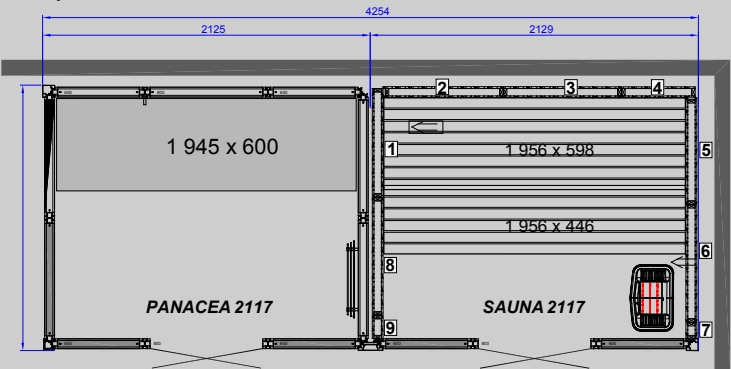
TWIN PANACEA 2117 Taille : 1 725 mm (p) x 4 254 mm (l)
