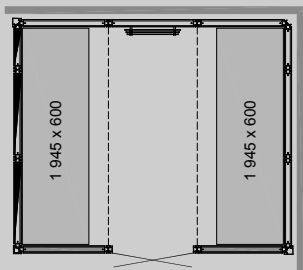
PANACEA 2521 2B Taille : 2 525 x 2 125 x 2 090 mm
