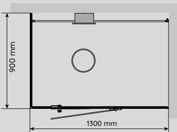
VISTA 130 GAUCHE Taille : 900 mm (p) x 1 300 mm (l)
