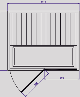
TYLÖSAND T-820 Taille : 1 013 mm (p) x 1 213 mm (l) Power : 1470W
