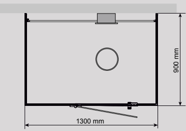
VISTA DCO 130 DROITE Taille : 900 mm (p) x 1 300 mm (l)
