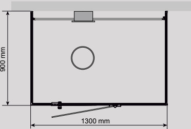
VISTA DCO 130 GAUCHE Maße: T 900 x B 1300 mm
