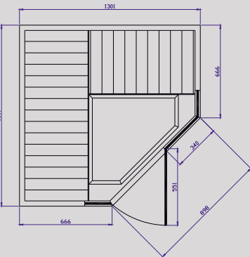
TYLÖSAND T-870 Taille : 1 301 mm (p) x 1 301 mm (l) Power : 1600W
